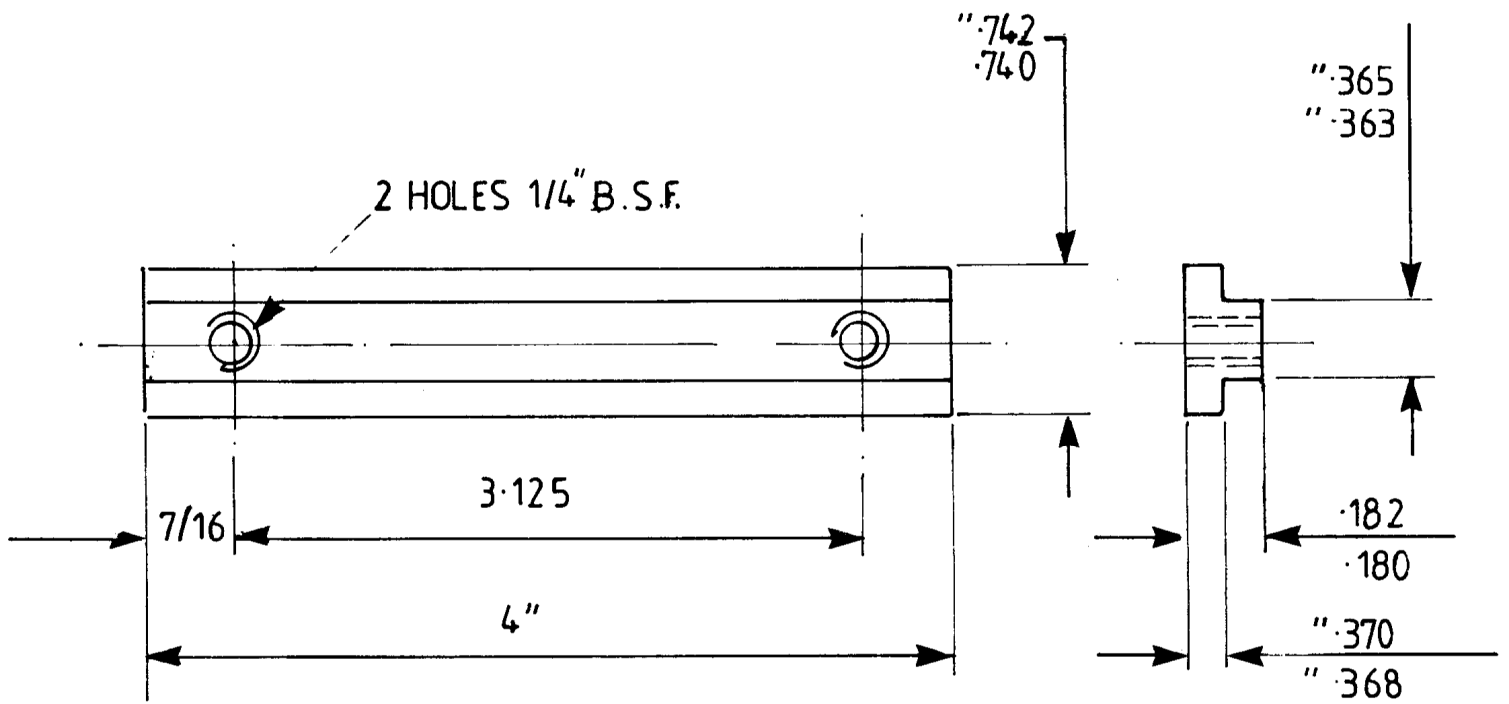
ITEM 10 TEE NUT MILD STEEL QTY 2.
