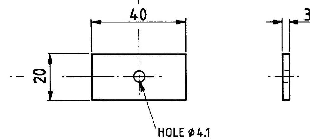
ITEM 10 DIE BLOCK MILD STEEL QTY 1
