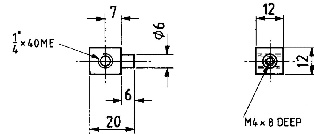
ITEM 10 DIE BLOCK MILD STEEL QTY 1
